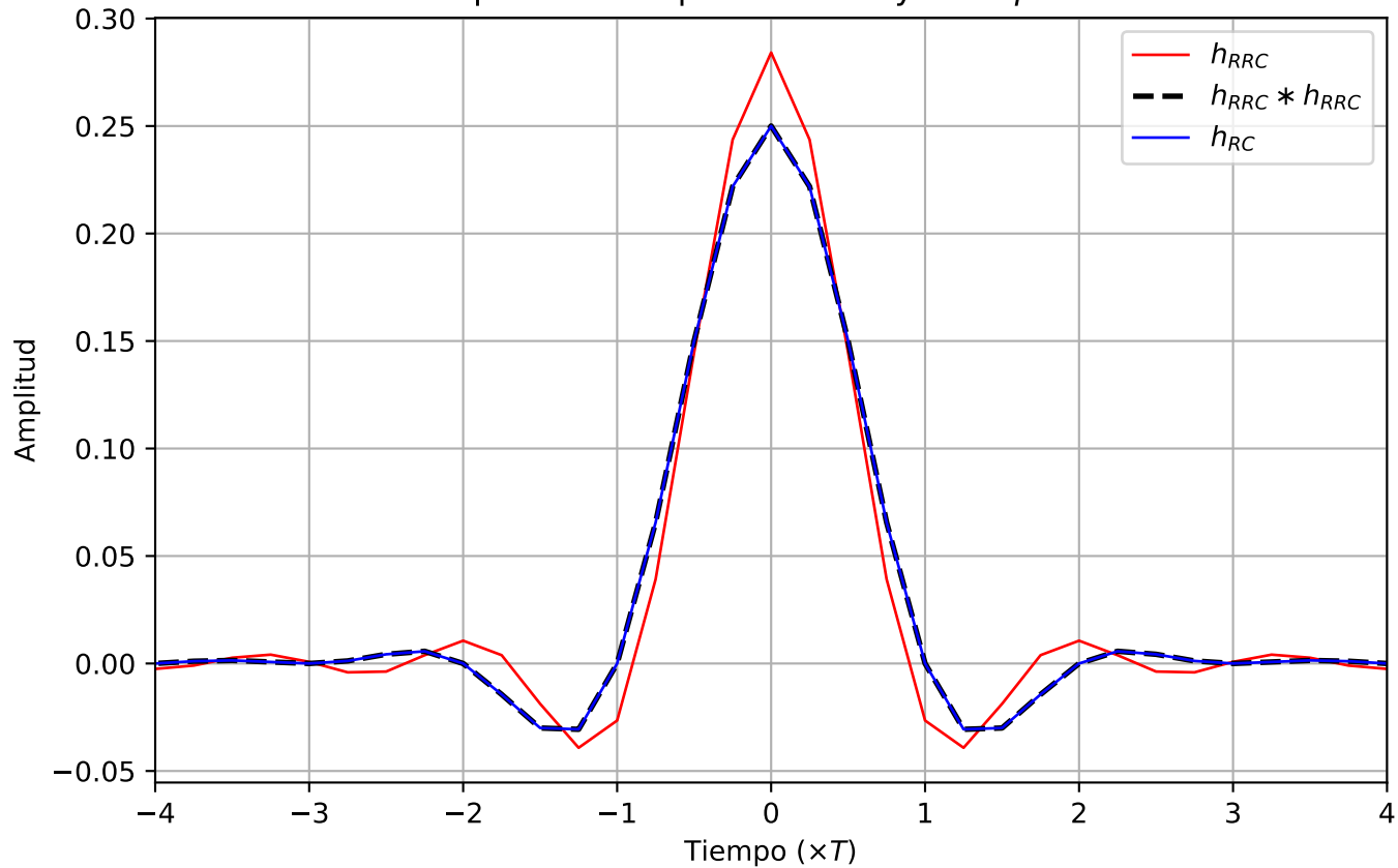
Respuesta al Impulso del RC y RRC. \beta = 0.5
